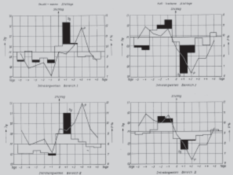
Illustration 6 : Synchronisation non fortuite d'ondes infra-longues et de cas de poliomyélite. Les barres noires montrent les jours où l'activité des sferics est faible (barres vers le bas) et ceux où l'activité est importante (barres vers le haut); les courbes superposées montrent le nombre de cas de poliomyélites recensés dans les années 50.
