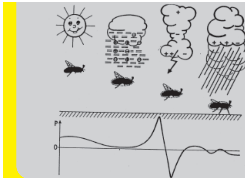
Illustration 2 : Schéma ci-dessus : La charge électrique des insectes se modifie typiquement en fonction des paramètres météorologiques. La courbe montre les modifications du champ électrique en fonction de la météorologie chez une abeille volant librement ; cette modification est schématisée dans le dessin en haut.
