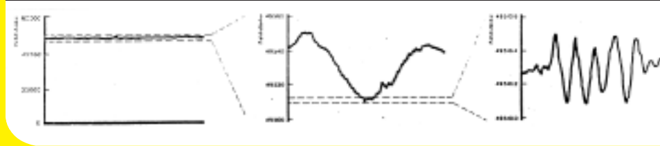
Illustration 22 : Variations du champ magnétique terrestre : sensibilité de la mesure respectivement augmentée du facteur 1000. On distingue les rythmes des journées et les micropulsations que les abeilles et autres organismes utilisent pour leur orientation dans l'espace et dans le temps.
