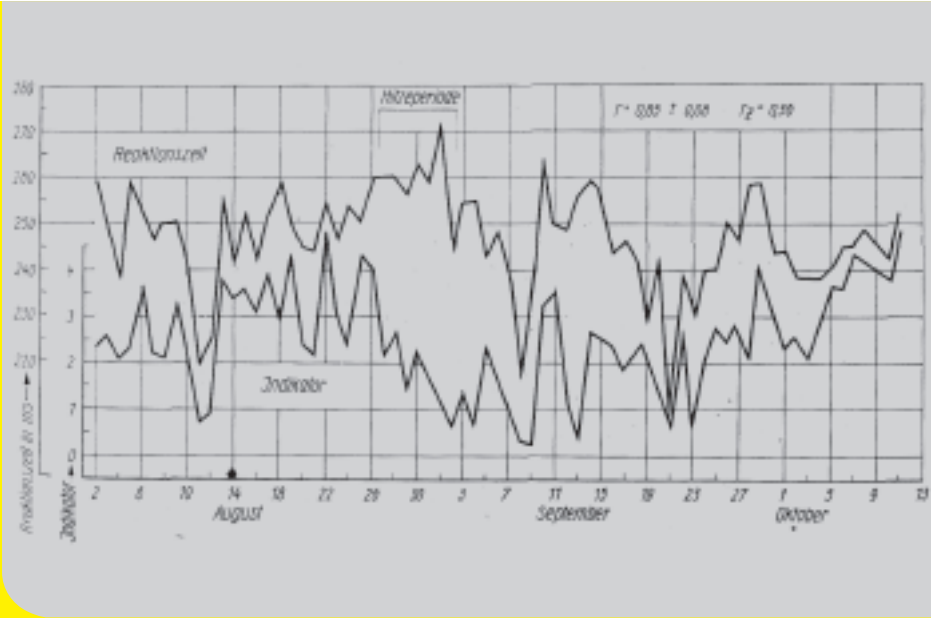
Illustration 5 La corrélation linéaire entre les activités des ondes infra longues électromagnétiques et le temps moyen de réaction chez les visiteurs d'une exposition n'est pas fortuite. Reiter, R. 1960 Meteorobiologie und Elektrizität der Atmosphäre. Akademische Verlagsges. Geest & Portig, Leipzig
