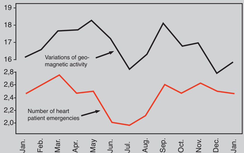
Illustration 7 : Moyenne mensuelle des hospitalisations quotidiennes en urgence pour infarctus du myocarde (courbe inférieure) et activité géomagnétique (courbe supérieure).
