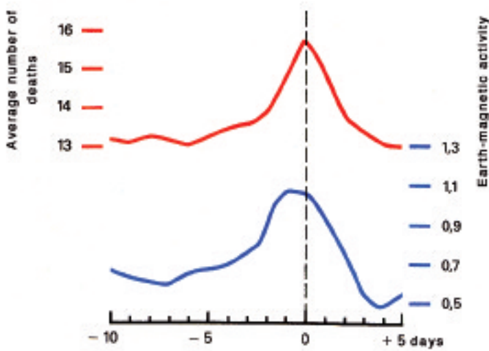
Illustration 8 : Tempêtes magnétiques (en bas) et mortalité due à des affections nerveuses et cardiovasculaires.
